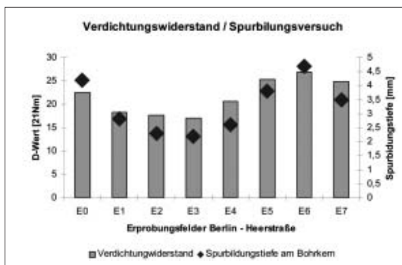
Abb. 3: Verdichtungswiderstand/Verformungsverhalten
